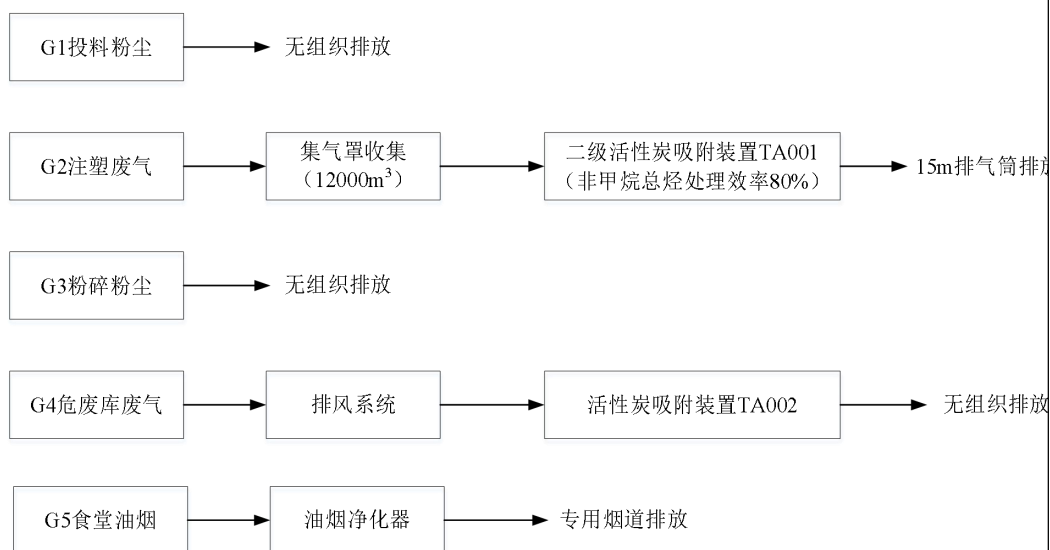
图4-1 全厂废气收集处理示意图
