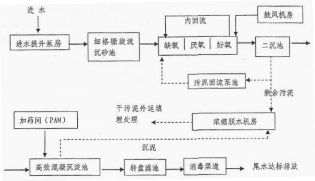
图 4-4 汤山污水处理厂工艺流程图
