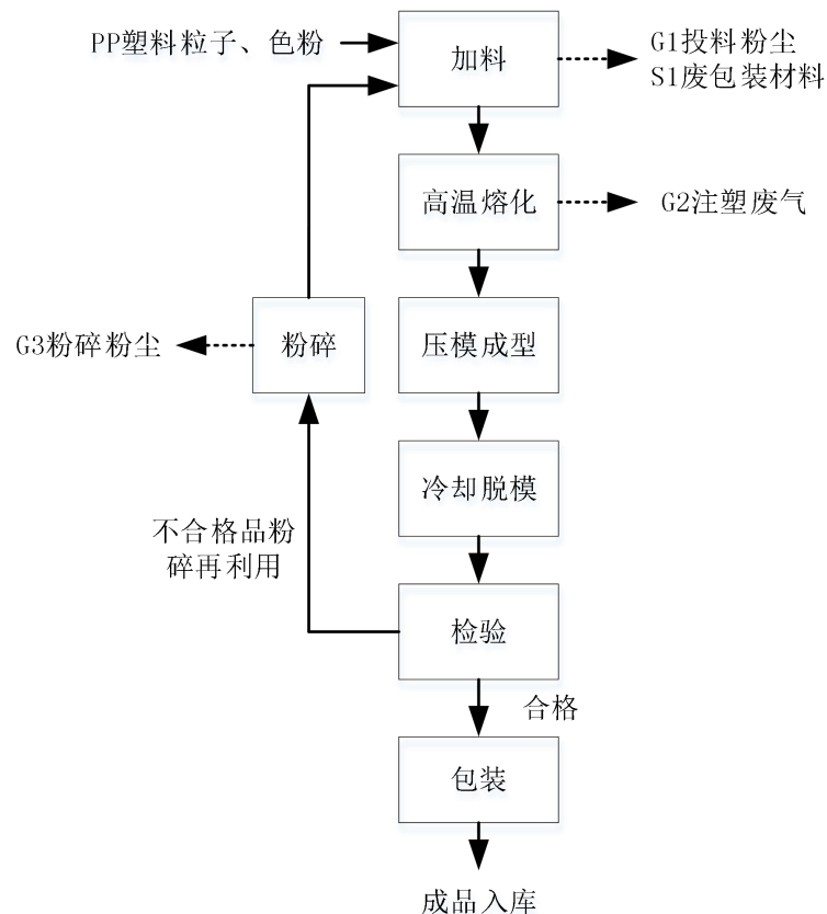
图 2-2 一次性塑料餐盒生产工艺流程及产污节点图
